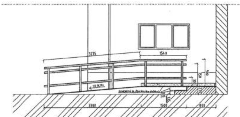
РЕЗЕРВНОЕ РАМПО А-А'
