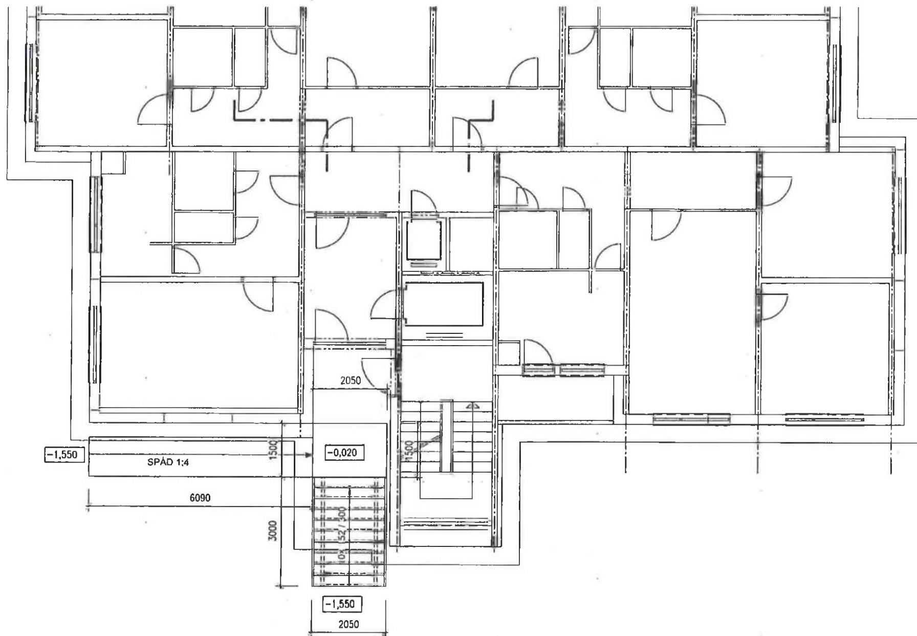
BALTSKÁ č.1 BRATISLAVA VSTUPNÁ RAMPA DO OBJEKTU PÓDORYS 1NP NOVÝ STAV VARIANT č.1 PODĽA ŽELANIA ZÁKAŽNÍKA
