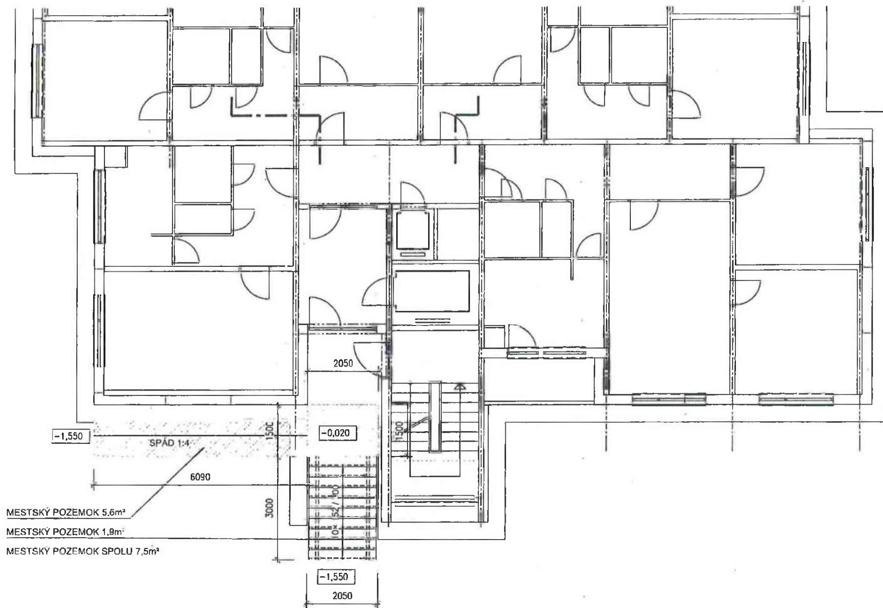
BALTSKÁ č.1 BRATISLAVA VSTUPNÁ RAMPA DO OBJEKTU PÔDORYS 1NP NOVÝ STAV VARIANT č.1 PI OCHY MESTSKÉHO POZEMKU
