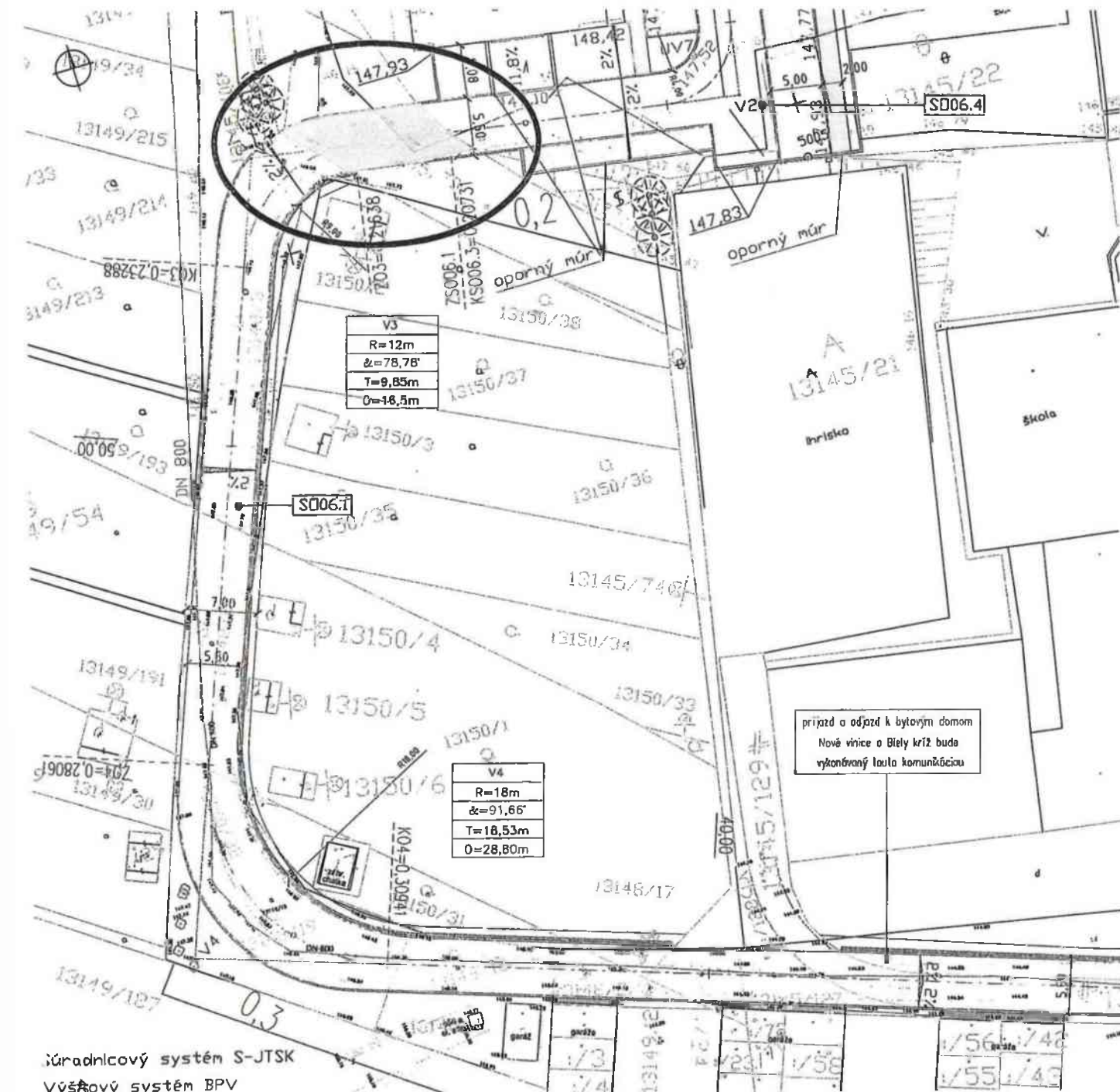
F.1 Miestna účelová komunikácia - napojenie na Skalickú cestu - SO-06.1
