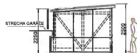
POHĽAD BOČNÝ
