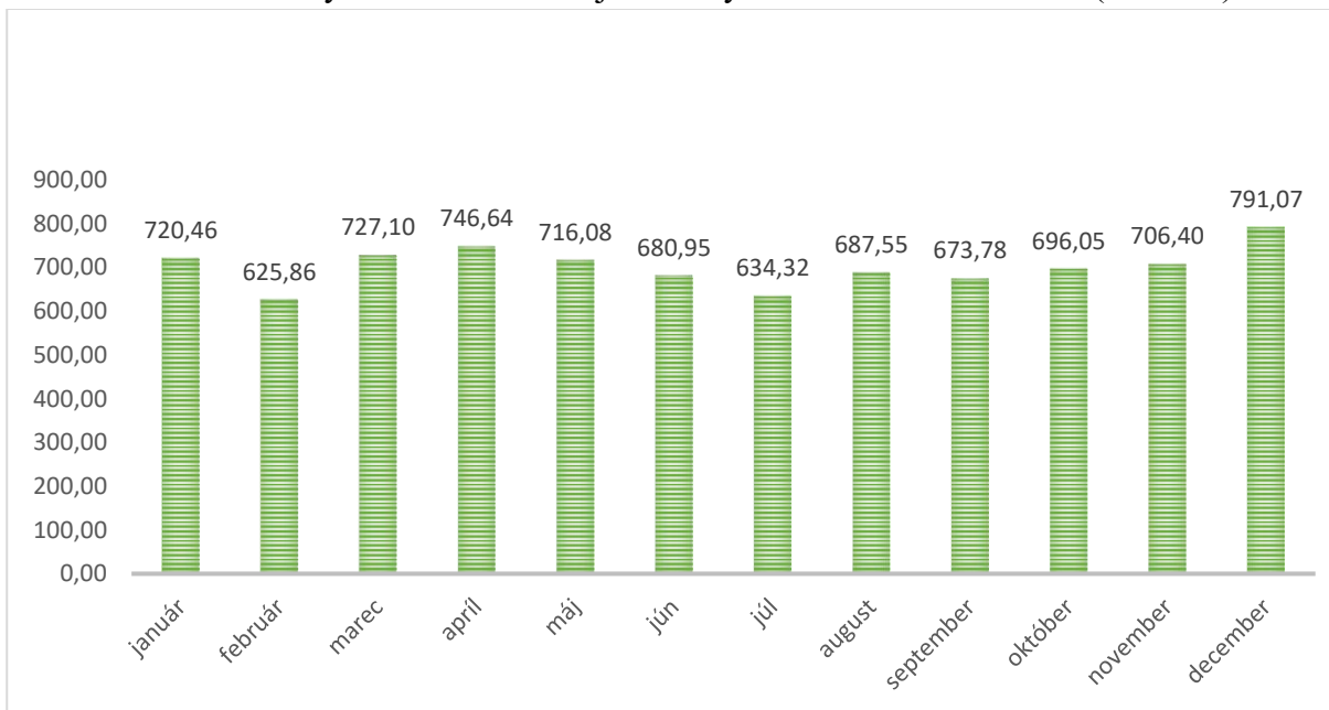
Graf č.12 Množstvo vyzbieraného skla v jednotlivých mesiacoch roka 2021 (mesiac/t)
