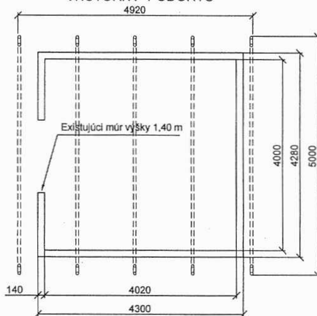
VNÚTORNÝ PÔDORYS
