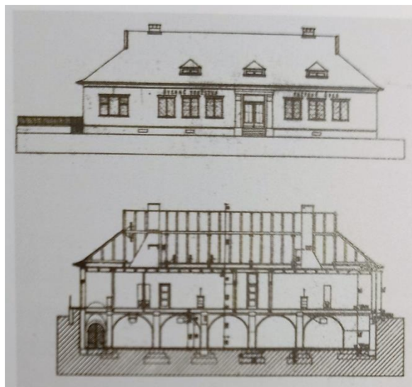
Pôvodný plán z r.1937
