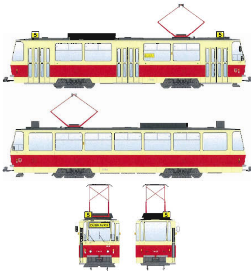
Obr. 10. Vizualizácia dráhového vozidla – električky typu T6A5/I
